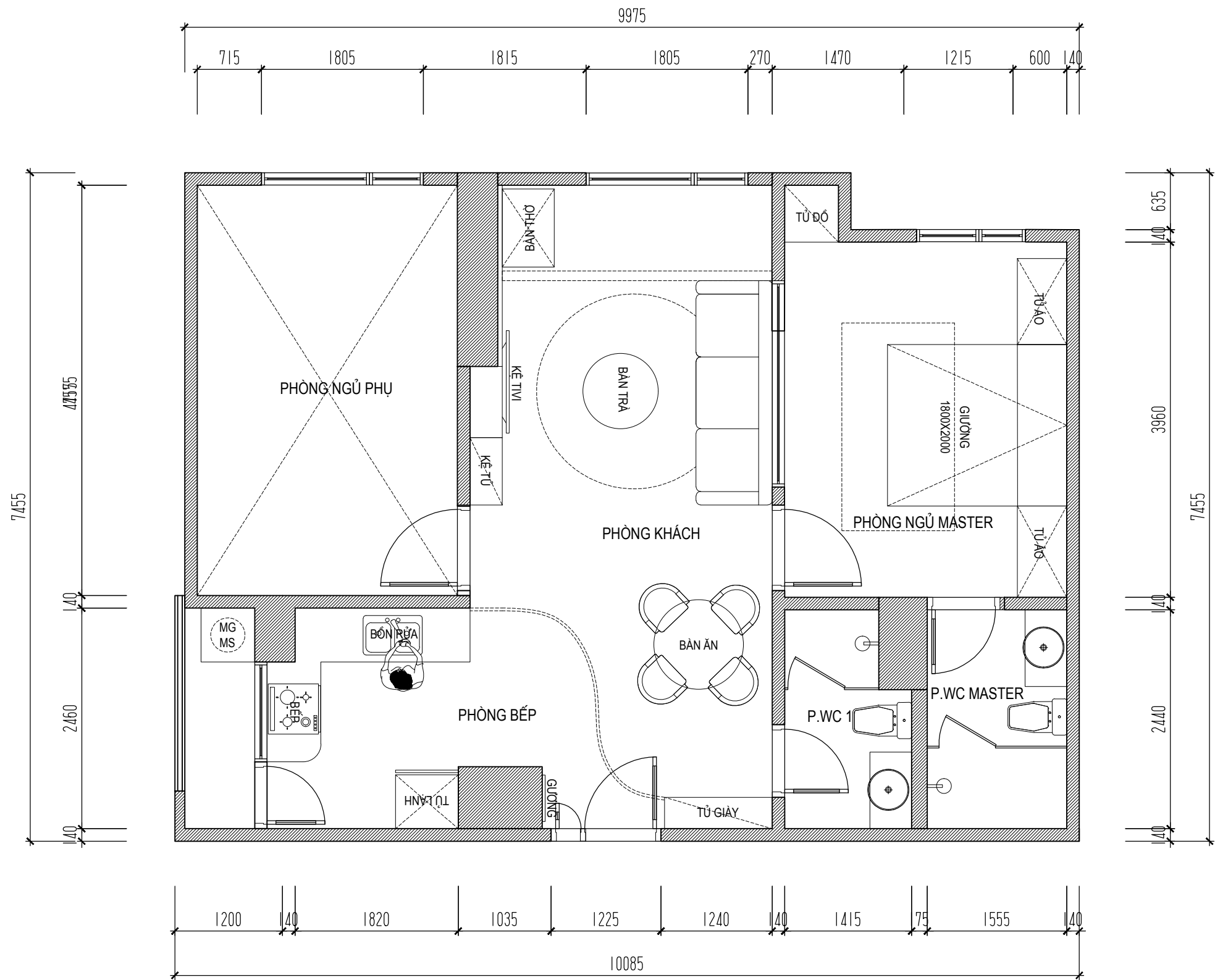
PHƯƠNG ÁN BỐ TRÍ MẶT BẰNG CĂN HỘ
